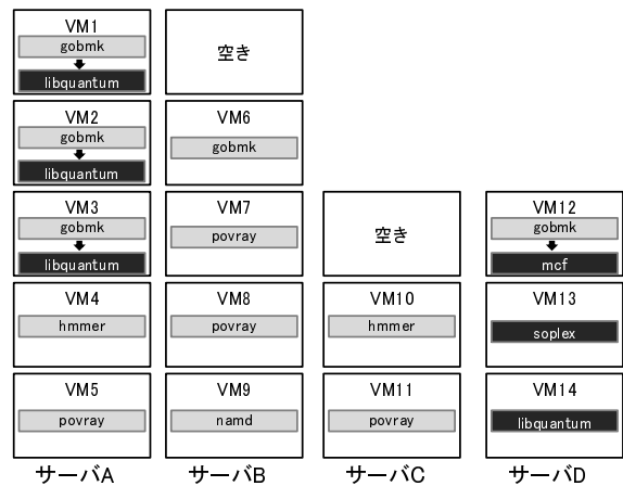
図 3: VM 上で実行するアプリケーションの特徴が変化する場合
