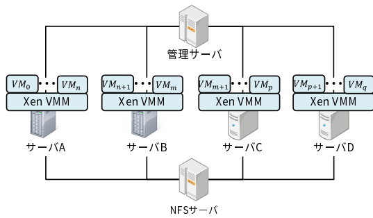
図 2: 作成した実験環境
