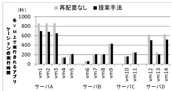
図 4: VM 上で実行するアプリケーションの特徴が変化する場合
